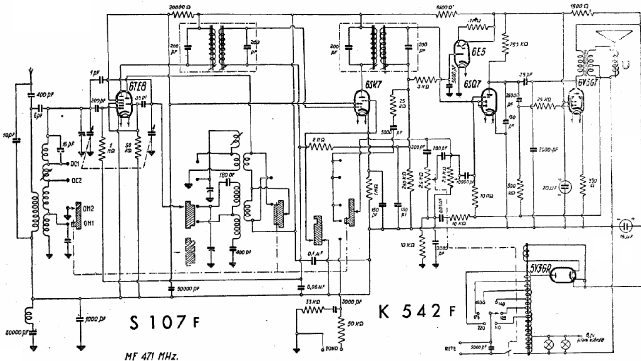
MAGNADINE RADIO - Mod. S 107 F e mod. Kennedy K 542 F - Onde medie divise e due gamme onde corte. Media frequenza 471 kc. Occhio magico. Reazione inversa dal secondario del trasformatore d'uscita. Potenza d'uscita indistorta 3,5 watt.
